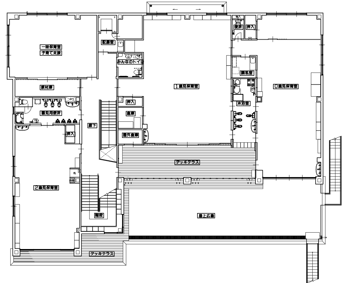
2階平面図
